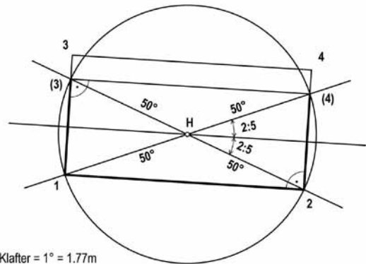
Abb. 3: Gründungsstadt Wiener Neustadt, Konstruktion des rechteckigen Hauptplatzes über ihre Diagonalen.
