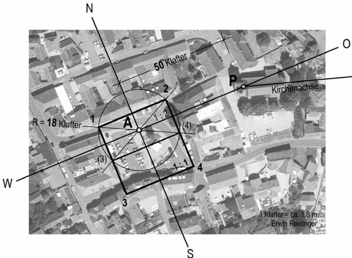
Abb. 11: Stadt Friedberg, Konstruktion des Hauptplatzes zur Bestimmung des Gründungspunktes A und des Verknüpfungspunktes mit der Kirche (Portalpunkt P) in geordneter Darstellung (Luftbild GIS Steiermark).
