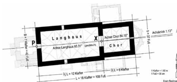
Abb. 16: Pfarrkirche Friedberg, Rekonstruktion des romanischen Grundrisses im historischen Maßsystem nach Auswertung der Detailvermessung (1 Klafter = 1.80 m, 1 Fuß = 0.30 m). Die Graustufe zeigt den heutigen Grundriss (Ansicht von Nordosten Abb. 15).
