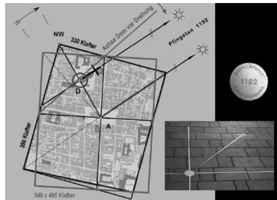
Abb. 2: Gründungsstadt Wiener Neustadt, Darstellung der Ausführung (330 x 390 Klafter, schwarz), die aus einem Grundrechteck (340 x 400 Klafter, rot) durch Drehung hervorgegangen ist. Der Gründungspunkt A sowie das Achsenkreuz mit dem Orientierungsstrahl (Sonnenaufgang Pfingsten 1192) sind auf dem Hauptplatz als „Vermessungsdenkmal“ markiert. Punkt D (blauer Ring) zeigt den Portalpunkt des Domes, der als Schnittpunkt von Achse Langhaus und Verdrehungsstrahl (A-NW) konstruiert wurde.
